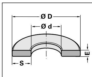
TOR-EF flache Ringkissen aus Elastomer/Gewebe max. Druck: 7 bar Ring cushion of elastomere/fabric, flat design max. pressure: 7 bar
