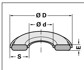
TOR-PF flache Ringkissen aus Polyurethan/Gewebe max. Druck: 0,5 bar Ring cushion of polyurethane/fabric, flat design max. pressure: 0,5 bar
