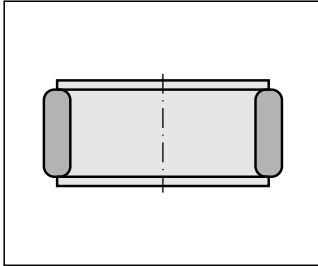
TOR-PH hohe Ringkissen aus Polyurethan/Gewebe max. Druck: 0,5 bar Seite 9-10 Ring cushion of polyurethane/fabric, high design max. pressure: 0,5 bar Page 9-10
