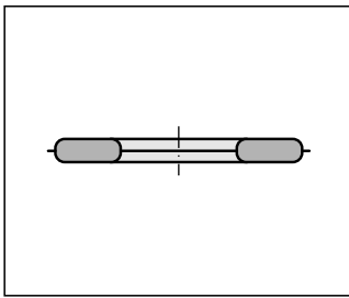
TOR-PF flache Ringkissen aus Polyurethan/Gewebe max. Druck: 0,5 bar Seite 9-10 Ring cushion of polyurethane/fabric, flat design max. pressure: 0,5 bar Page 9-10
