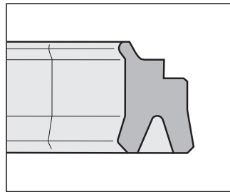
1PL Dicht-Abstreifer für verdrehgesicherte Pneumatikzylinder, Seite 14 Seal Wiper for rotation protected pneumatic cylinders, page 14
