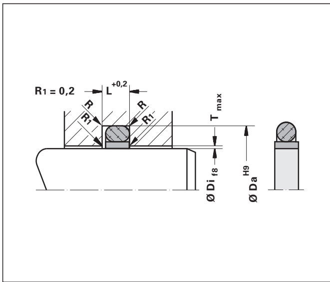
PTFE-Gleitdichtungssatz 1G0 PTFE Glide Seal Set 1G0
